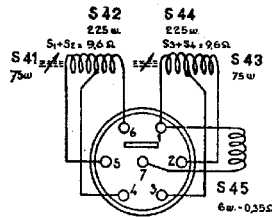
MF.SPOEL I GK 563 74
