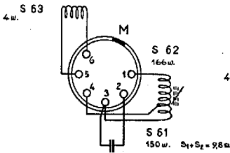
MF.SPOEL III GK 563 76
