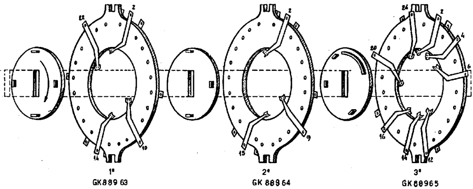
DE DRIE SEGMENTEN DER GOLFBEREIKSCHAKELAAR, VAN VOREN GEZIEN
