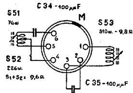
MF.SPOEL II GK 563 75
