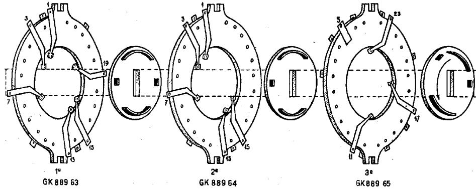
DE DRIE SEGMENTEN DER GOLFBEREIKSCHAKELAAR, VAN ACHTEREN GEZIEN
